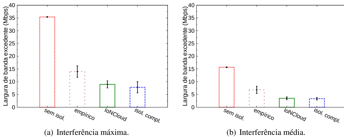
Figura 4. Interferência entre tráfegos, medida pela banda excedente à reservada.
